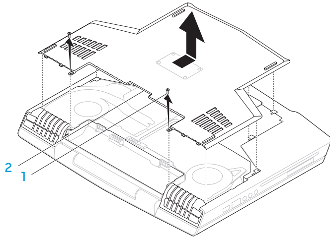
1 Schrauben (2)
